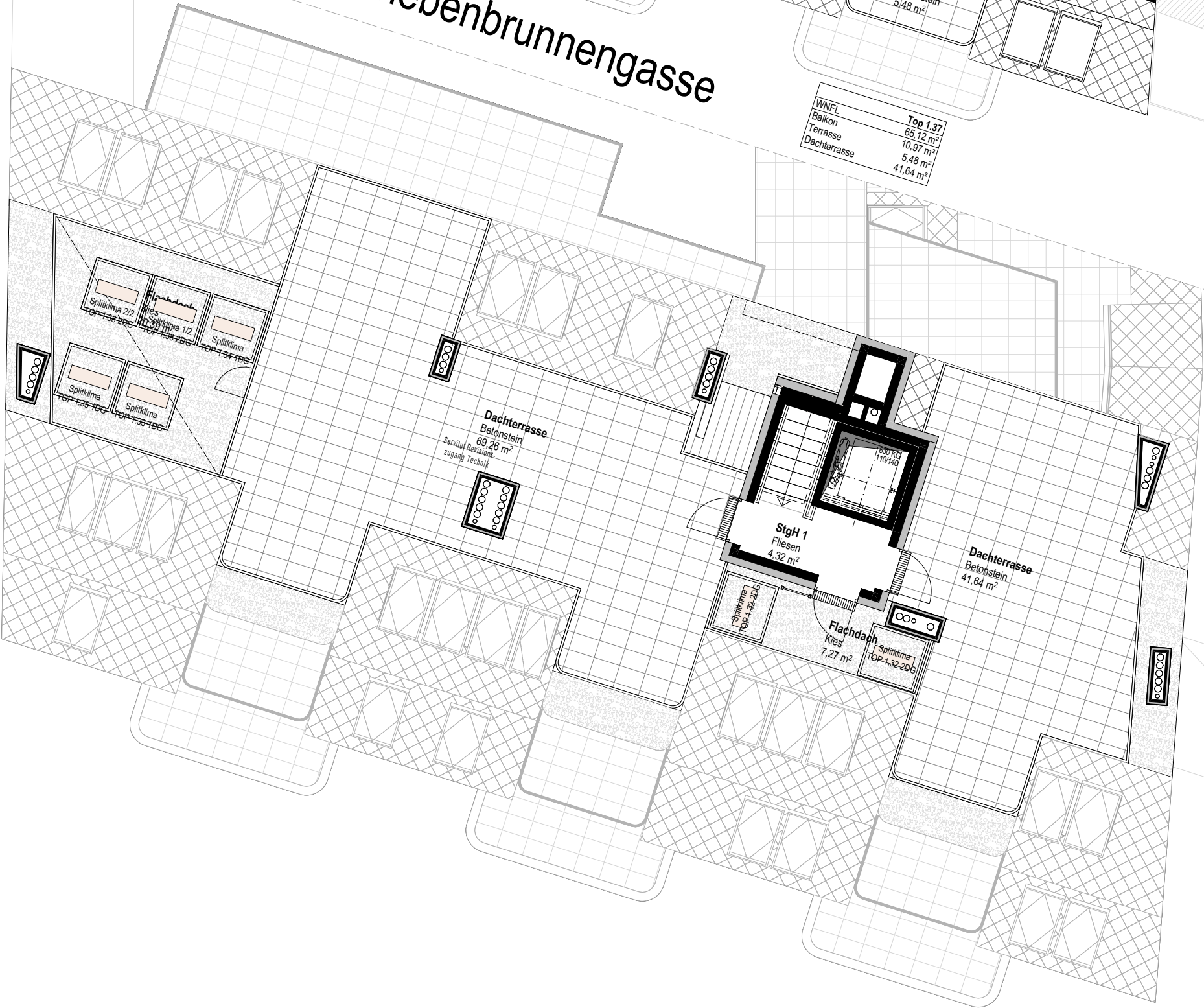
Dachdraufsicht Straßentrakt ü. 2.DG
